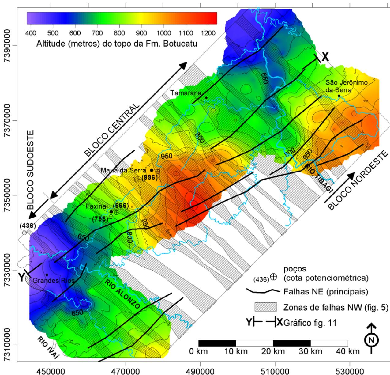
Figura 9: Mapa de contorno do topo da Formação Botucatu com sobreposição das ZFs NW da figura 5 e das falhas N40-60E mais contínuas nos fotolaneamentos da figura 4.
