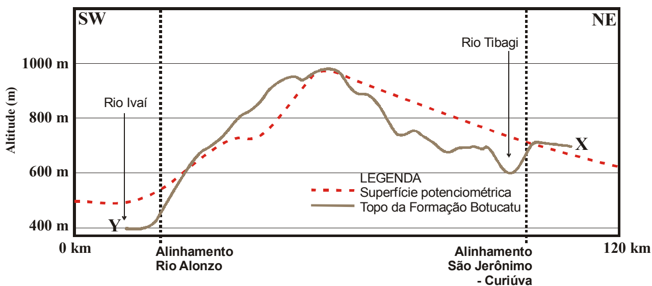
Figura 11: Gráficos mostrando a comparação entre as curvas altimétricas de potencimetria e dos contornos de topo da Formação Botucatu, num perfil transversal às estruturas NW (localização: vide figura 8)
